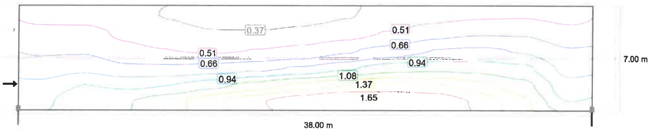
Observator 1: Densitatea luminii la instalația nouă [cd/m 2 ] (Linii Isolux)
